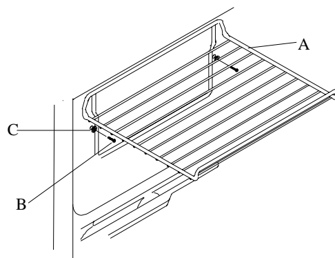
A. Grille utilitaire à glaçons B. Vis
