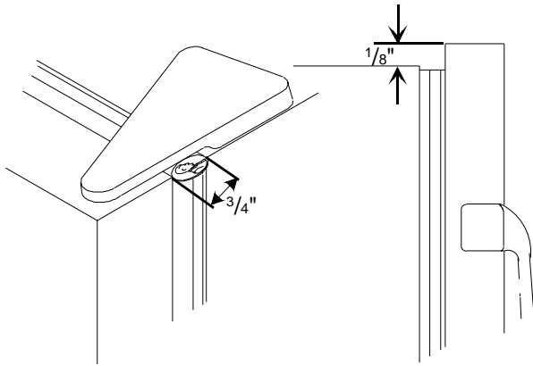
Door spacing
