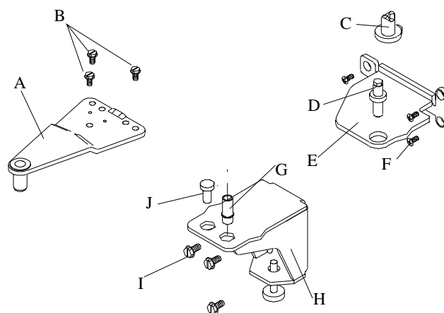
A. Charnière supérieure B. Vis de \frac{5}{16} " po (8 mm) C. Ferme-porte D. Axe de la charnière centrale E. Charnière centrale F. Vis cruciformes G. Axe de la charnière inférieure H. Charnière inférieure I. Vis de \frac{3}{8} " po (10 mm) J. Bonde en plastique
